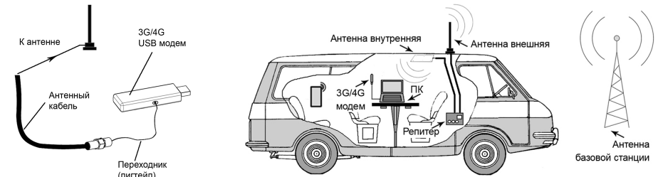
Схема 1 – Подключение антенны к USB модему
